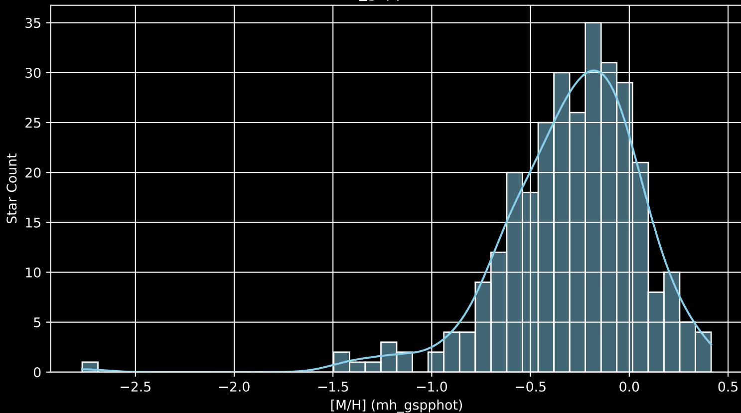
GALAH DR4 Field: [70] [M/H] (mh_gspphot) (n= 303)
