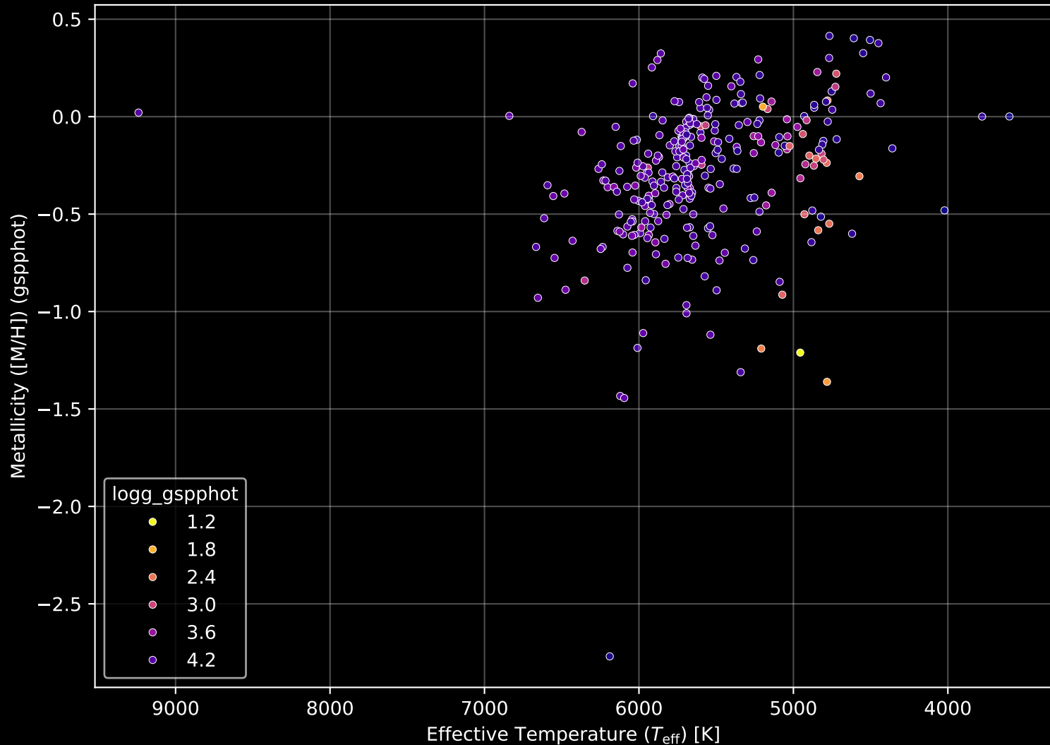
GALAH DR4 Field: [70] Stellar Population Parameters (n= 303)
